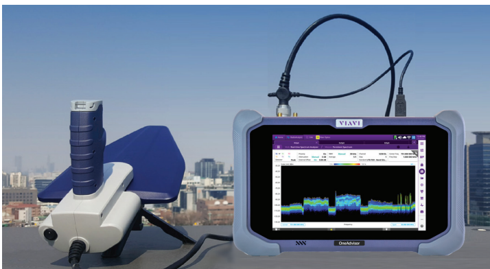
An den CellAdvisor angeschlossener AntennaAdvisor
