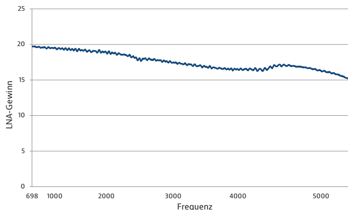
Gewinn-Kennlinie des Peilgeräts AntennaAdvisor
