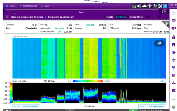
Получение спектрограмм в реальном времени с помощью анализатора OneAdvisor 800
